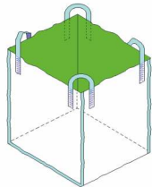
überkreuzte Vernähung
